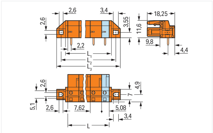
Dimensions en mm L = (\text{nombre pôles} - 1) \times \text{pas} + 5,08 \text{ mm} L1 = L + 3 \text{ mm} L2 = L + 8,8 \text{ mm} L3 = L + 14,8 \text{ mm} Connecteurs femelles de 2 à 3 pôles – seulement 1 crochet d'arrêt
