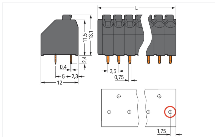
Dimensions en mm L = (nombre de pôles x pas) + 1,5 mm (Cercle rouge) première broche à souder devant à droite
