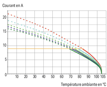
2-, 4-, 6-, 12-, 24-pôles — Courant nominal de la borne
