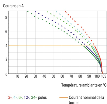
Courbe d'intensité maximale admissible Pas 2,5 mm / section de conducteur 0,5 mm 2 « s » Selon l'exemple de : EN 60512-5-2 / facteur de réduction 1
