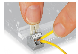
Connexion/Déconnexion des conducteurs – Actionnement manuel – Série 256.
