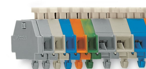
Barrette à bornes avec pieds de fixation à encliquer, pour épaisseur de tôle 0,6 ... 1,2 mm, diamètre de trou de fixation Ø 3,5 mm (aussi pour rail aluminium 210-154 ou avec pied de montage 209-120 sur rail DIN 35)
