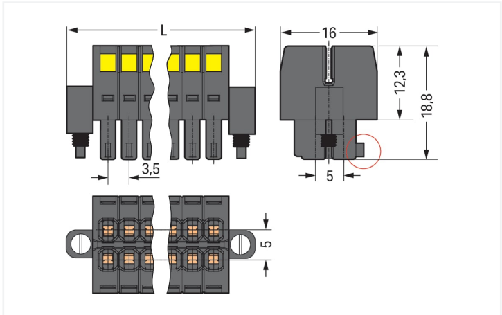
Dimensions en mm L = [(nombre de pôles/2) – 1] x pas + 13,6 mm (cercle rouge) tige de codage
