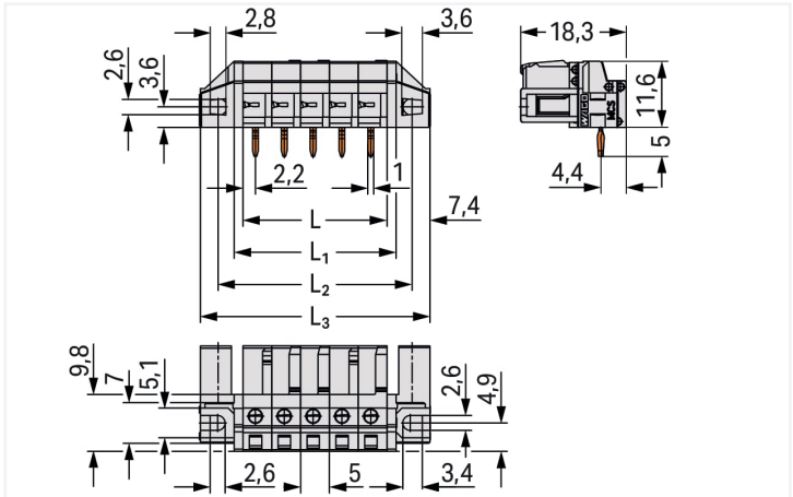
Dimensions en mm L = nombre de pôles x pas L1 = L + 3 mm L2 = L + 8,8 mm L3 = L + 14,8 mm Connecteurs femelles à 2 pôles – seulement 1 crochet d'arrêt
