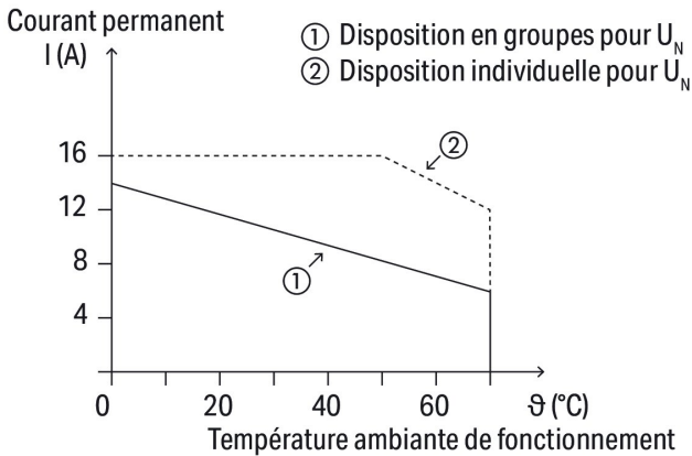
Courbe d'intensité maximale admissible
