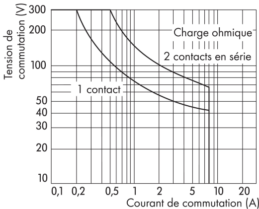
Courbe de limite de charge
