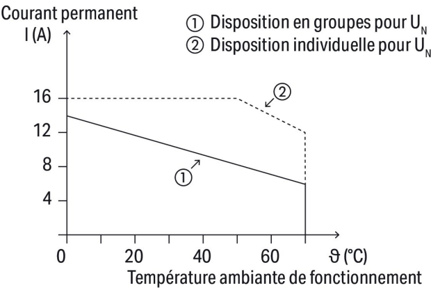
Courbe d'intensité maximale admissible
