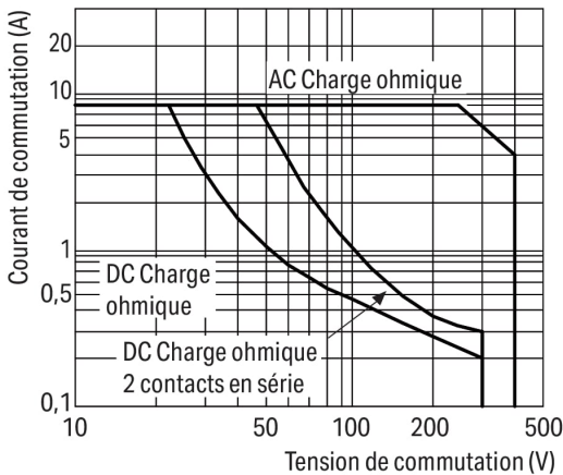
Courbe de limite de charge
