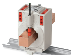
Montage sur barre de cuivre
