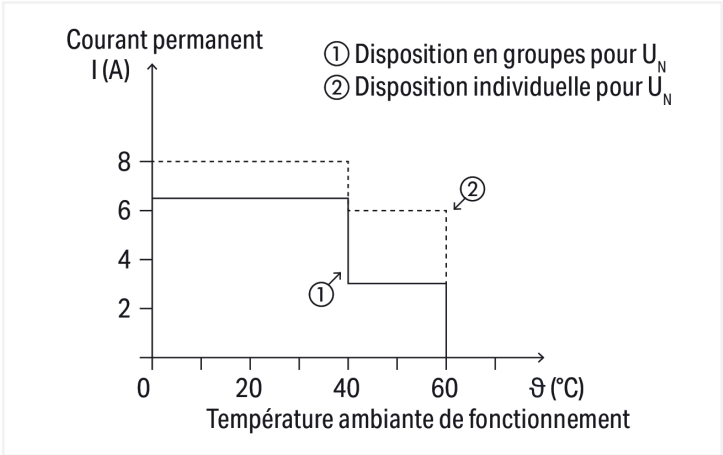
Courbe d'intensité maximale admissible UL
