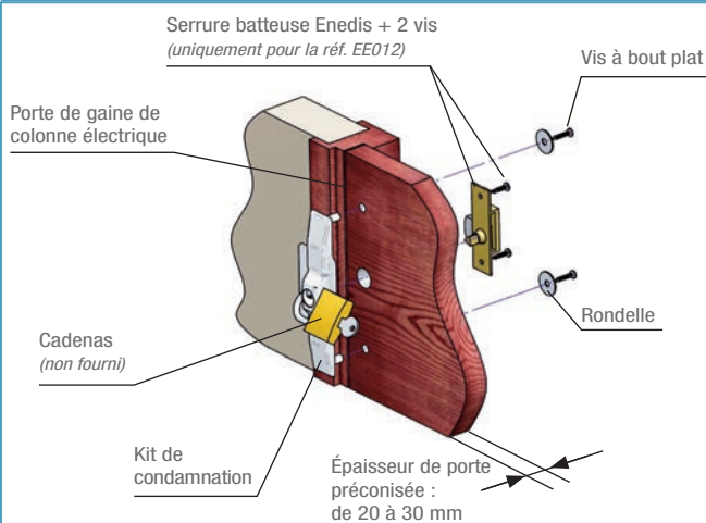
Avec serrure (EE012)
