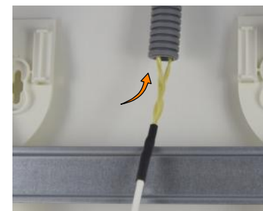
Pour un kit avec câble intérieur et/ou extérieur type L1081, L1082, L1083, L1084 ou L1088 : Poser le câble optique dans le conduit à l'aide d'une aiguille de tirage (conduit ø20 mini pour kit précâblé et conduit ø25 mini pour kit préconnectorisé).
