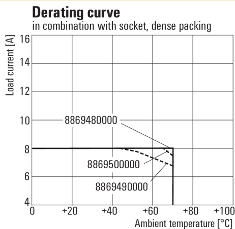
Courbe de dérating
