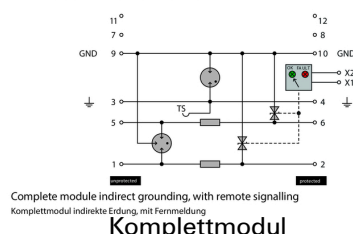
Komplettmodul
