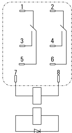
Vue des broches par dessous
