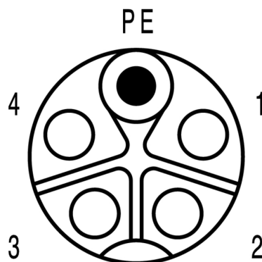
Socket
