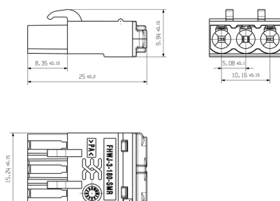
Steckverbinder Bauform 5 Connector type 5
