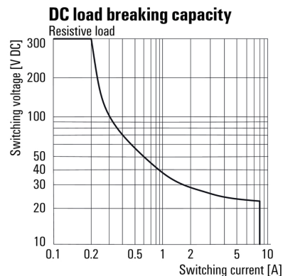
Courbe de charge limite DC Charge résistive
